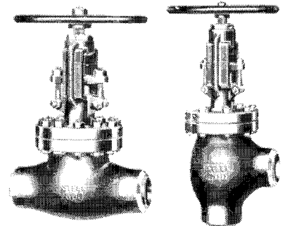
Buttweld Ends Globe 300LB 014301 600LB 016301 900LB 017301 1500LB 019301 Angle 300LB 014401 600LB 016401 900LB 017401 1500LB 019401
