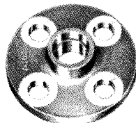
Flange 150 ANSI 605170 300 ANSI 605570 150 NAVY 605175 250 NAVY 605181
