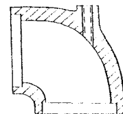
V&D Ell 513302
