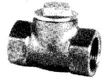
JIS Thread Check 5K JIS-B-2015 940505 10K JIS-B-2025 940510
